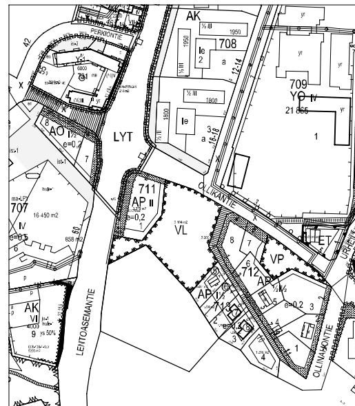
ASEMAKAAVA 1:2000
