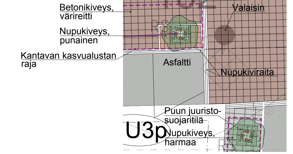
OTE 2 1:200
