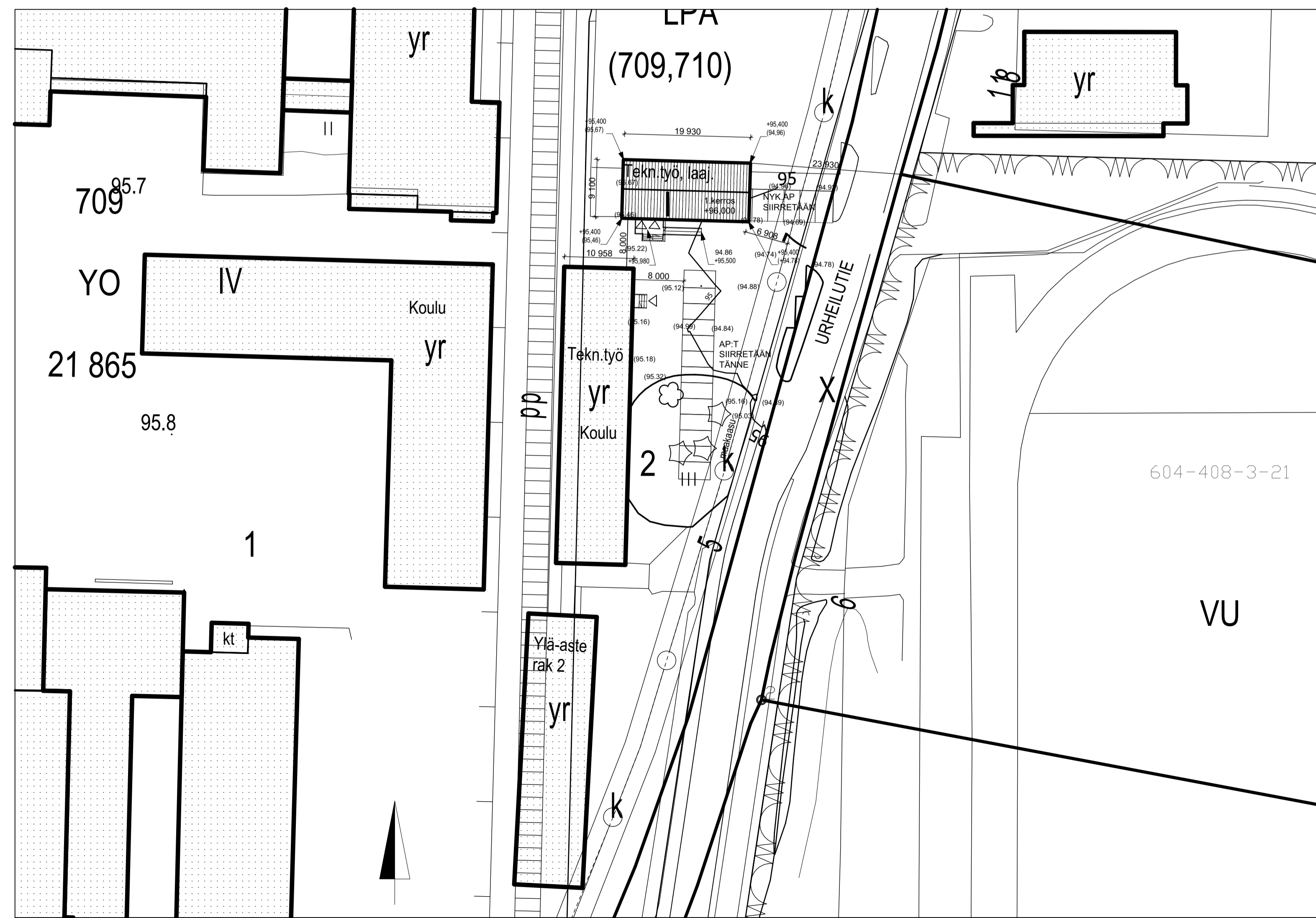
ASEMAPIIRUSTUSOTE 1:500
